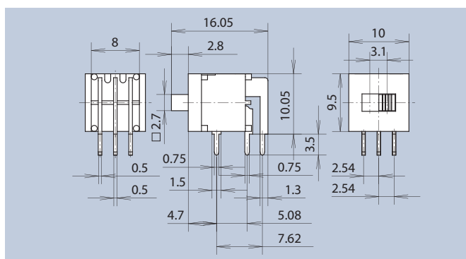
2259.1832 · 2-polig / 2 pole
