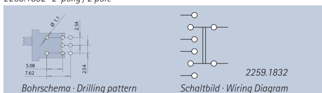
2259.1832 · 2-polig / 2 pole
