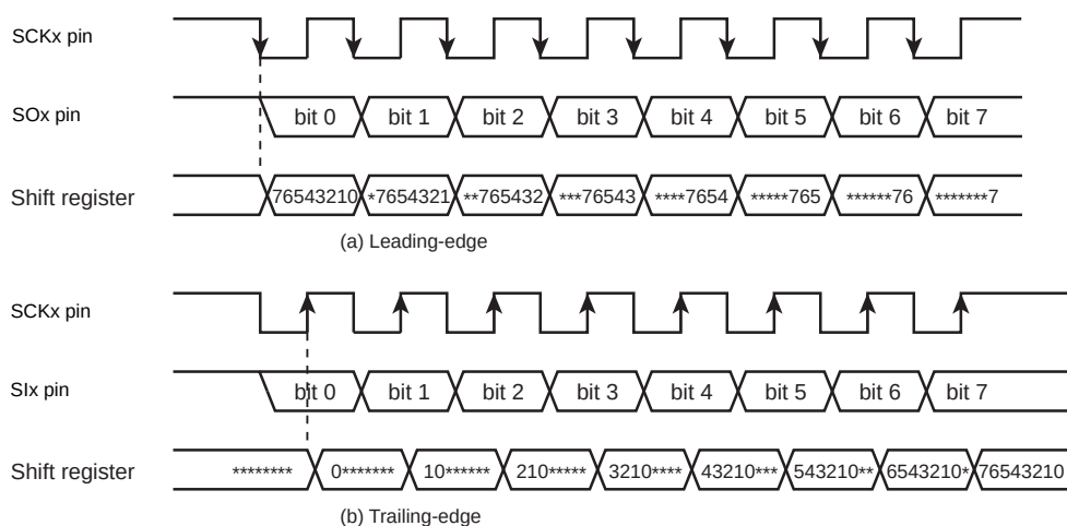
Figure 15-17 Shift Edge
