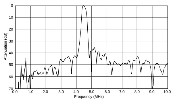
SFSRA4M50CF00-B0
