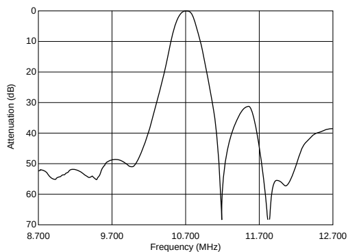
SFELF10M7GAXA-B0
