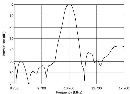
SFELF10M7GALM-B0
