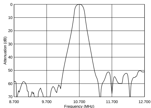
SFELF10M7GA0G-B0
