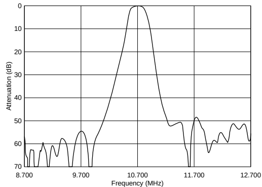
SFELF10M7FA0G-B0
