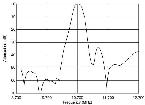
SFELF10M7GALP03-B0
