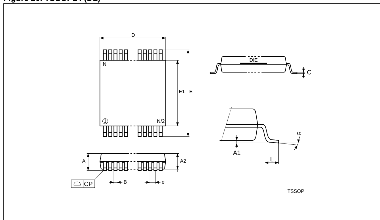
Figure 20. TSSOP14 (DL)
