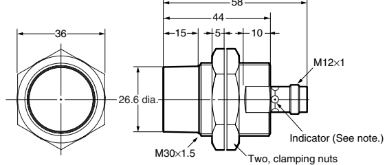
E2A-M30KN20-M1-□□/E2A-S30KN20-M1-□
