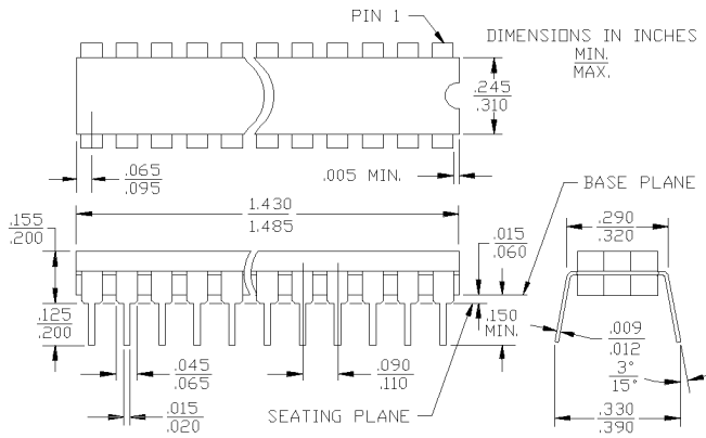
28-Lead (300-Mil) CerDIP D22 MIL-STD-1835 D-15 Config.A
