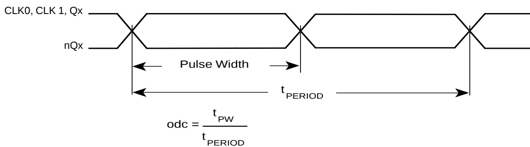
FIGURE 7 - odc & t_{PERIOD}
