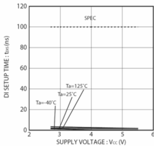
Figure 18. DI setup time t_{DIS}
