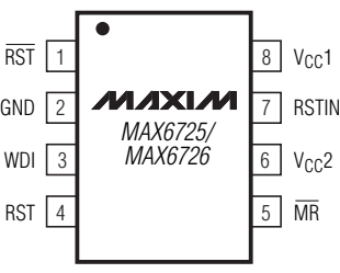
SOT23-8
