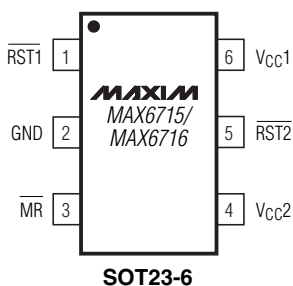
SOT23-6
