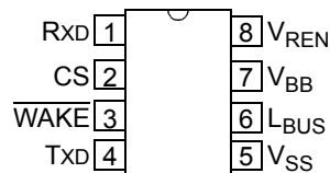
MCP2003B SOIC
