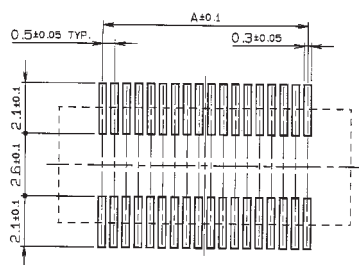
基板取り付け寸法 MOUNTING LAYOUT
