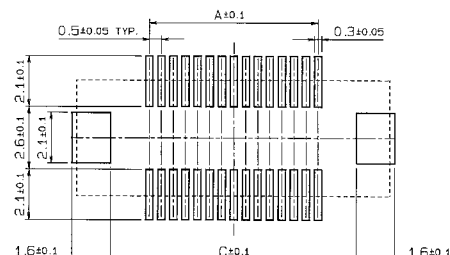
基板取付け寸法 MOUNTING LAYOUT
