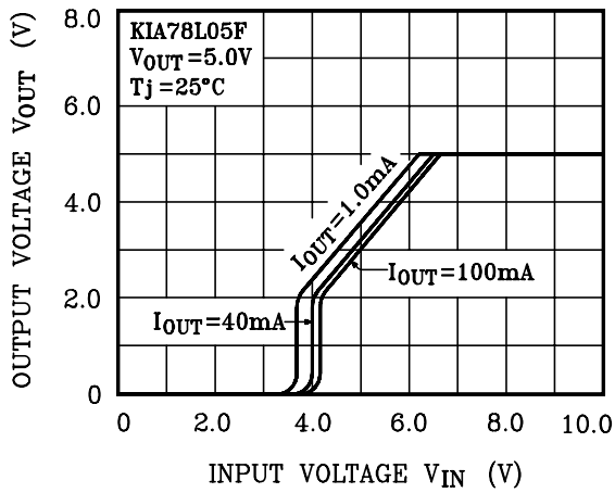
V_{OUT} - V_{IN}
