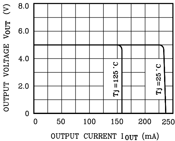
V_{OUT} - I_{OUT}
