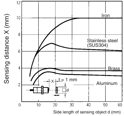
E2E-CR8□□
