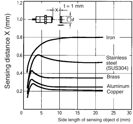
E2E-CR8□□
