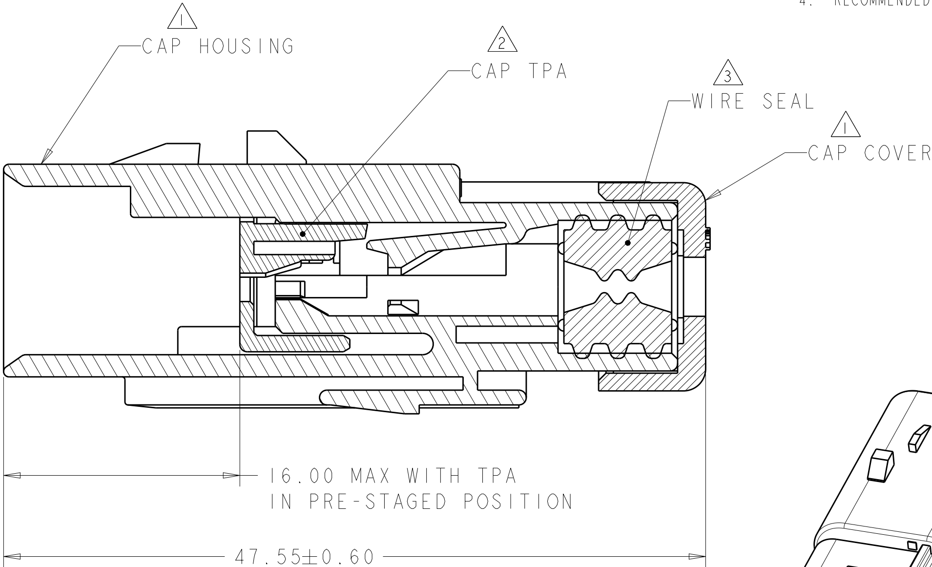
SECTION A-A
