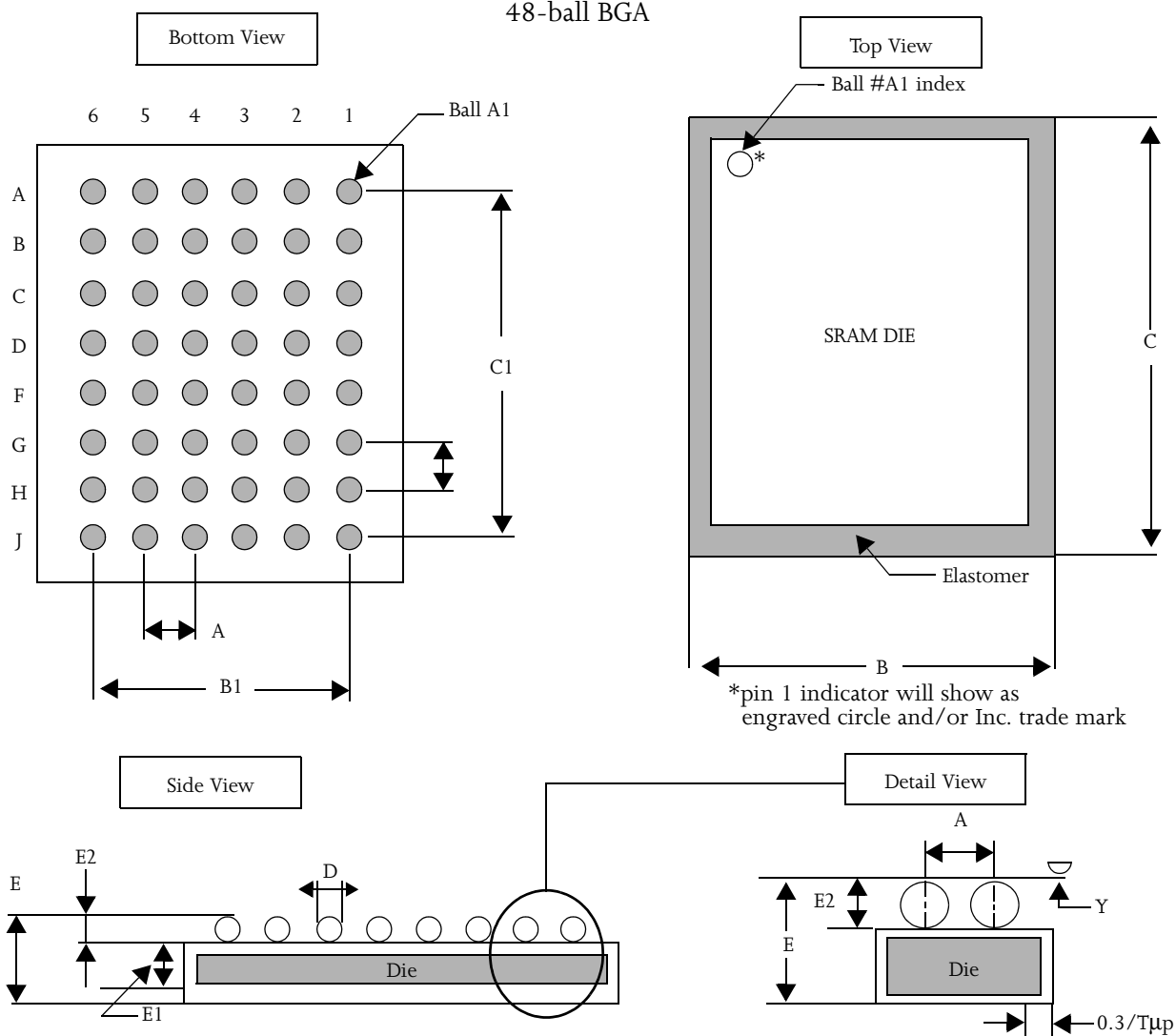
48-ball BGA
