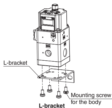
L-bracket
