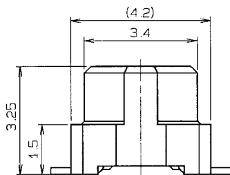
吸着テープ位置 POSITION OF VACUUM TAPE
