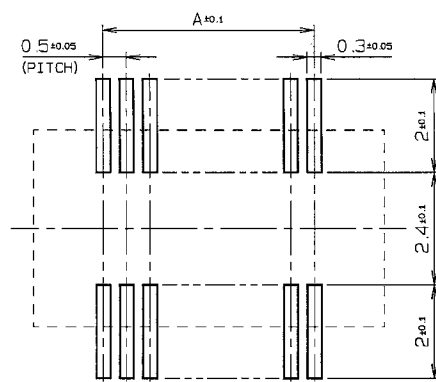
推奨基板レイアウト RECOMMENDED P.C. BOARD LAYOUT
