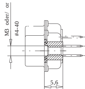
Schnitt A-A / cross section A-A
