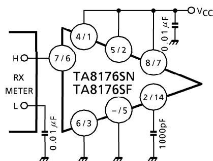
Pin⑦ / ⑥ input impedance
