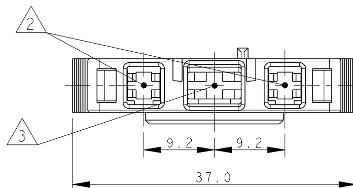
HOUSING (BLOCCHETTO)
