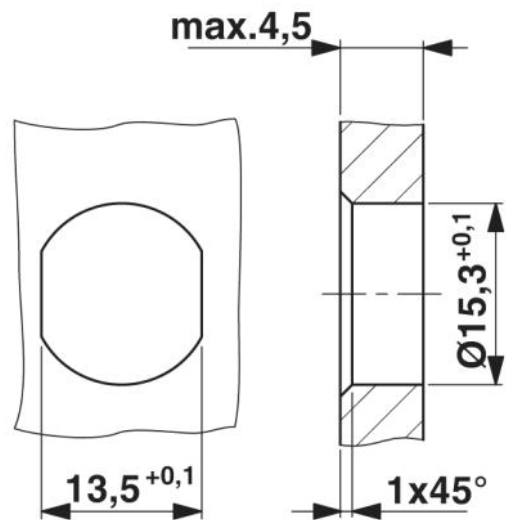
Montageausschnitt mit Verdrehsschutz für PG9-Gewinde
