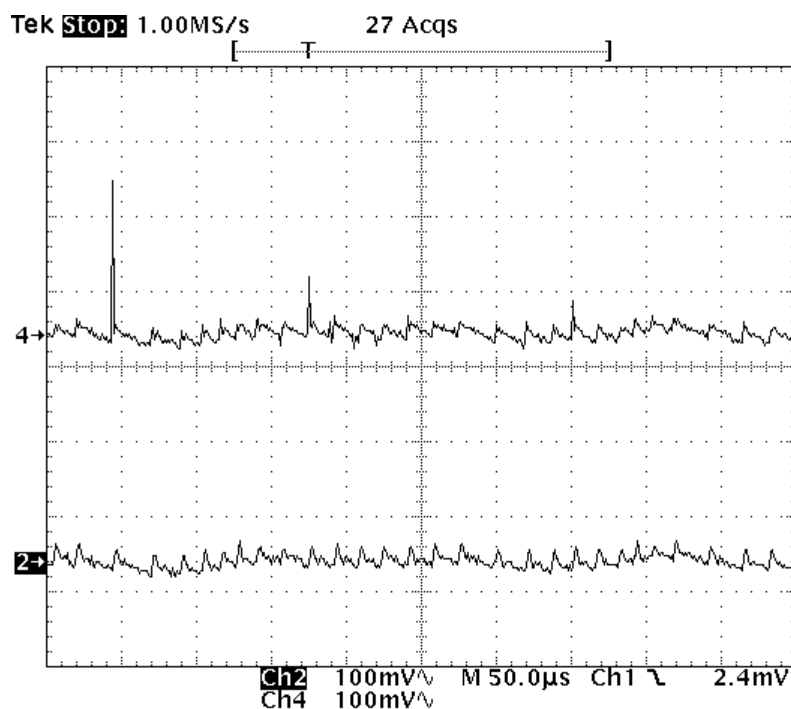
Figure 12. 0.6-A to 0.1-A Load Step
