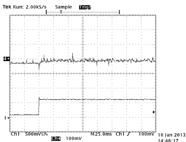
Figure 10. 0.6-A to 0.1-A Load Step
