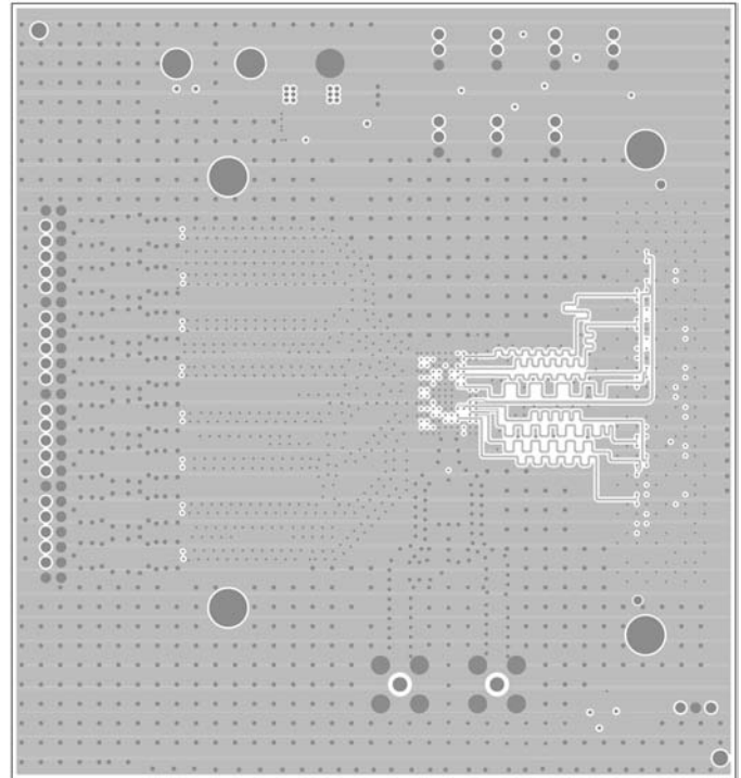
Inner Layer 5
