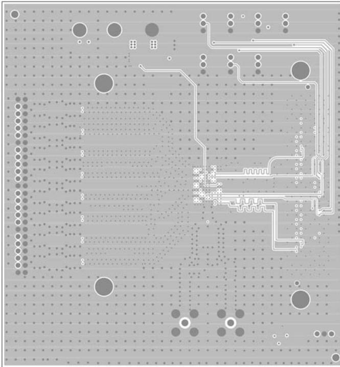
Inner Layer 4
