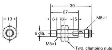
E2A-S08KN04-M5-□□
