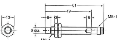
E2A-S08LN04-M5-□□
