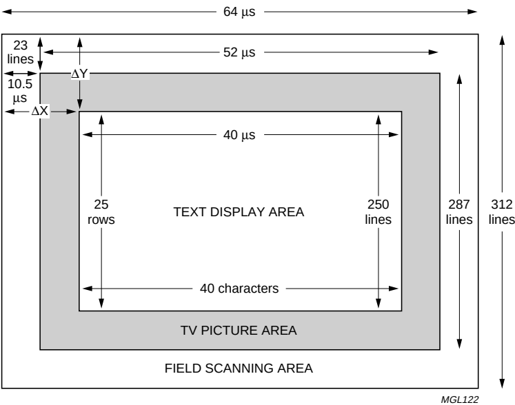
Fig.3 625 display format.
