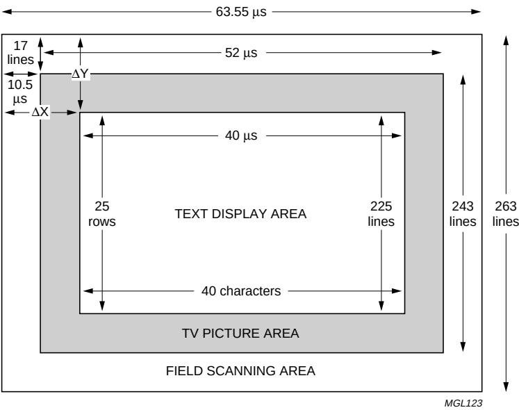
Fig.4 525 display format.
