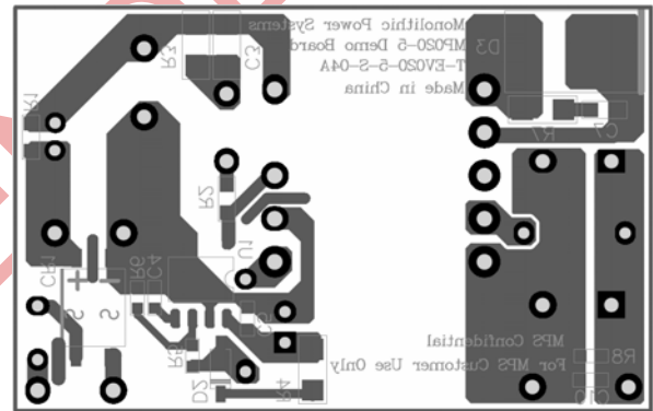
Bottom Layer
