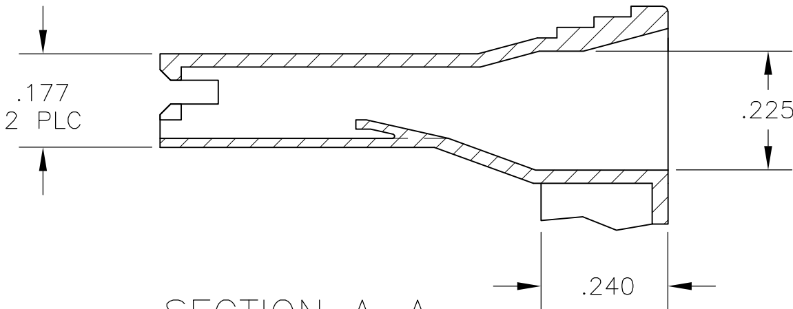
SECTION A-A
