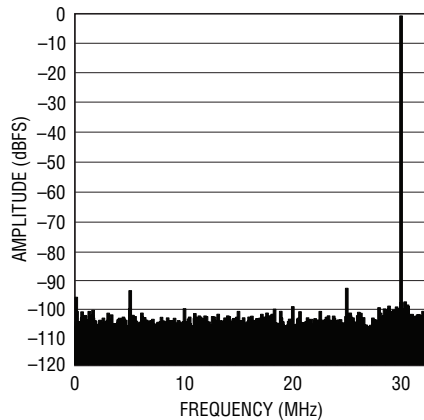
LTC2265-14: 8k Point FFT, f_{IN} = 30\text{MHz} , -1\text{dBFS} , 65\text{Mps}
