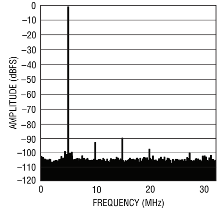
LTC2265-14: 8k Point FFT, f_{IN} = 5\text{MHz} , -1\text{dBFS} , 65\text{Mps}
