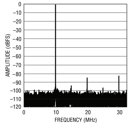
LTC2265-14: 8k Point FFT, f_{IN} = 140\text{MHz} , -1\text{dBFS} , 65\text{Mps}
