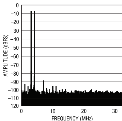
LTC2265-14: 8k Point 2-Tone FFT, f_{IN} = 68\text{MHz} , 69\text{MHz} , -1\text{dBFS} , 65\text{Mps}
