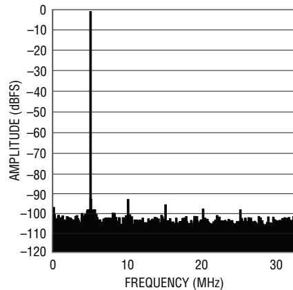
LTC2265-14: 8k Point FFT, f_{IN} = 70\text{MHz} , -1\text{dBFS} , 65\text{Mps}
