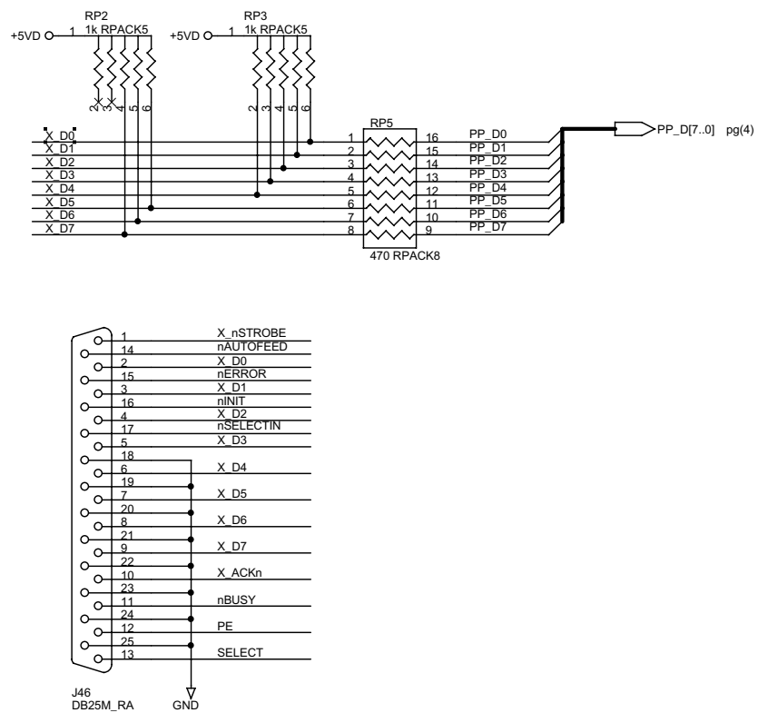
Figure 27. UDSP - Parallel Port Interface
