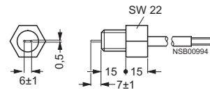
Einpilige Bügelelektrode 3UG32 07-1B
