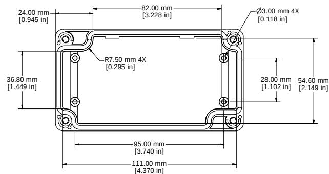
LID - INSIDE
