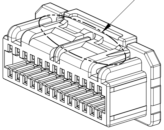
26-32CKT. ロック形状 LOCK SHAPE OF 26-32P
