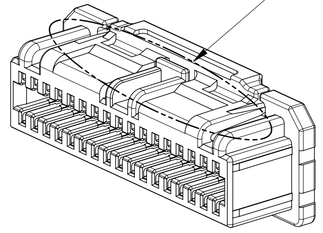
34-42CKT. ロック形状 LOCK SHAPE OF 34-42P
