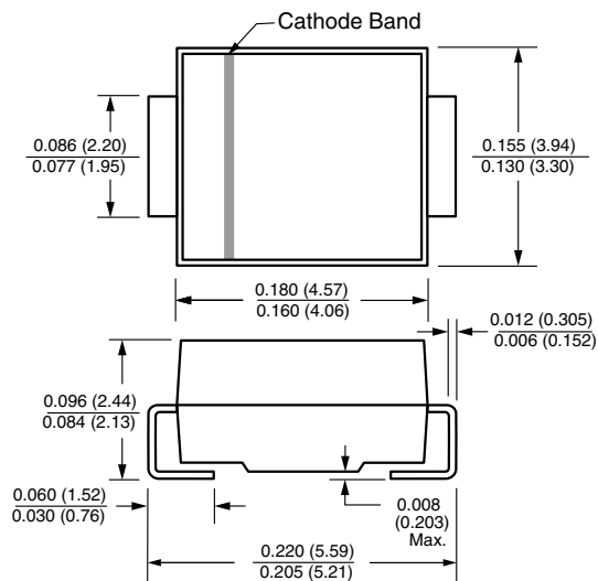
DO-214AA (SMBJ)
