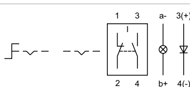
Wiring diagram 20
