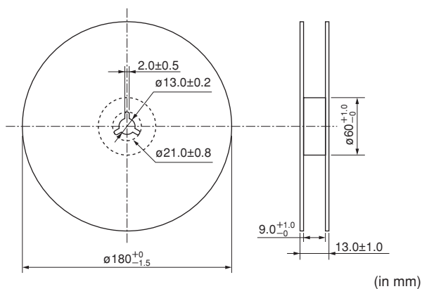
Reel Dimensions
