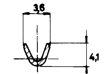
SECCION B-B
