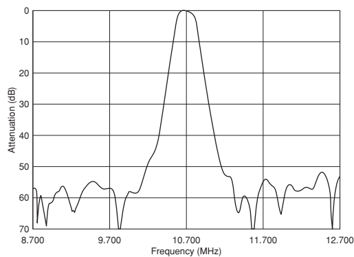
SFELF10M7GA00-B0
