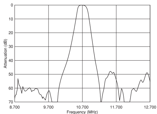
SFELF10M7FAB0-B0
