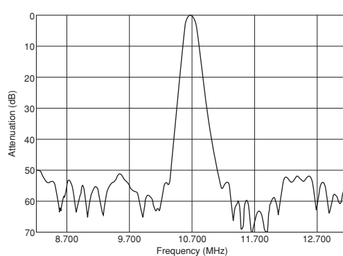
SFELF10M7JAB0-B0
