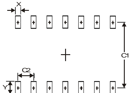
SO-14
