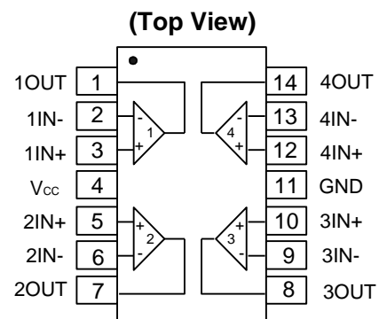
SO-14/TSSOP-14
