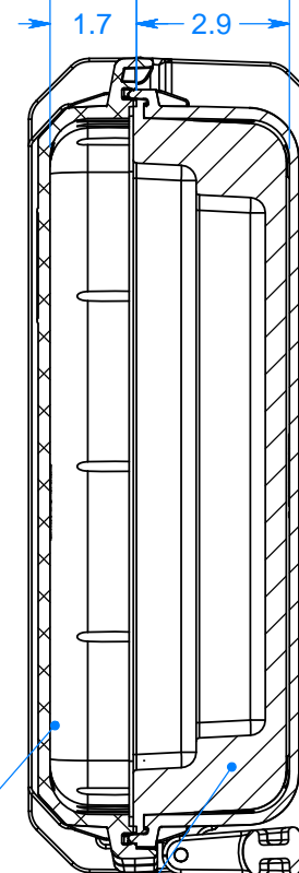
SECTION A-A
