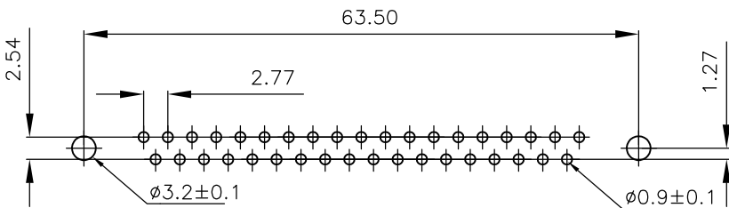
P.C.B. LAYOUT
