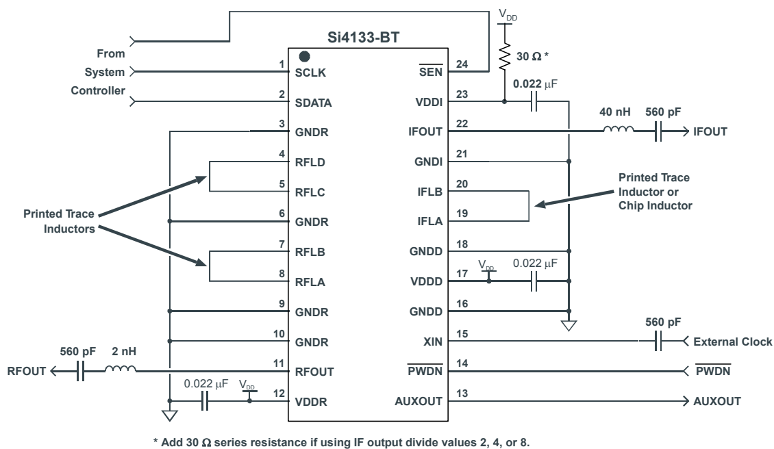
Figure 13. Si4133-BT
