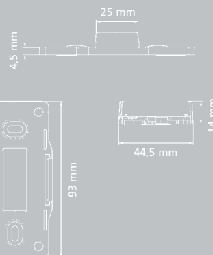
Wandhalterung 1813578
