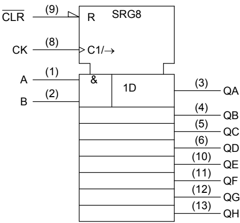
論理図
