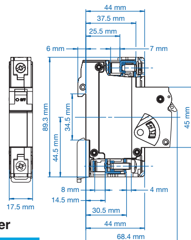
Dimensions N63UM, FxxUM.
