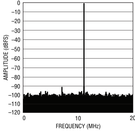
LTC2171-12: 8k Point FFT, f_{IN} = 69\text{MHz} , -1\text{dBFS} , 40\text{MSPS}
