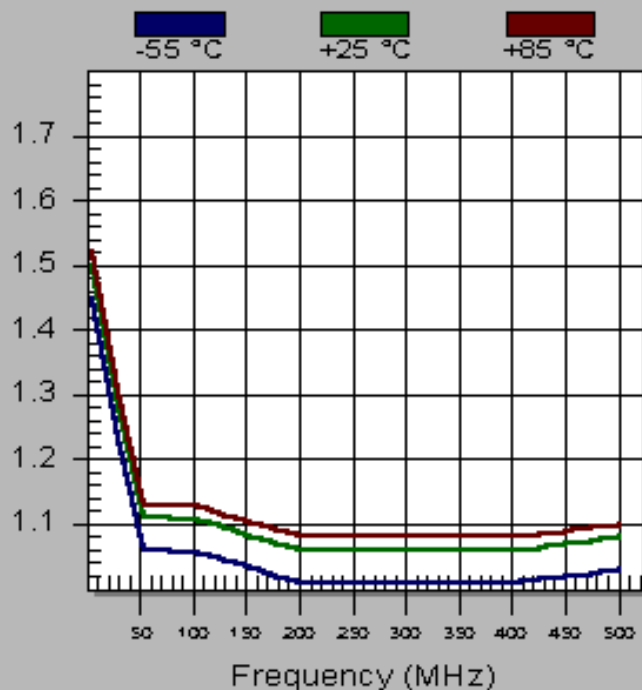
TM6520 Output VSWR
