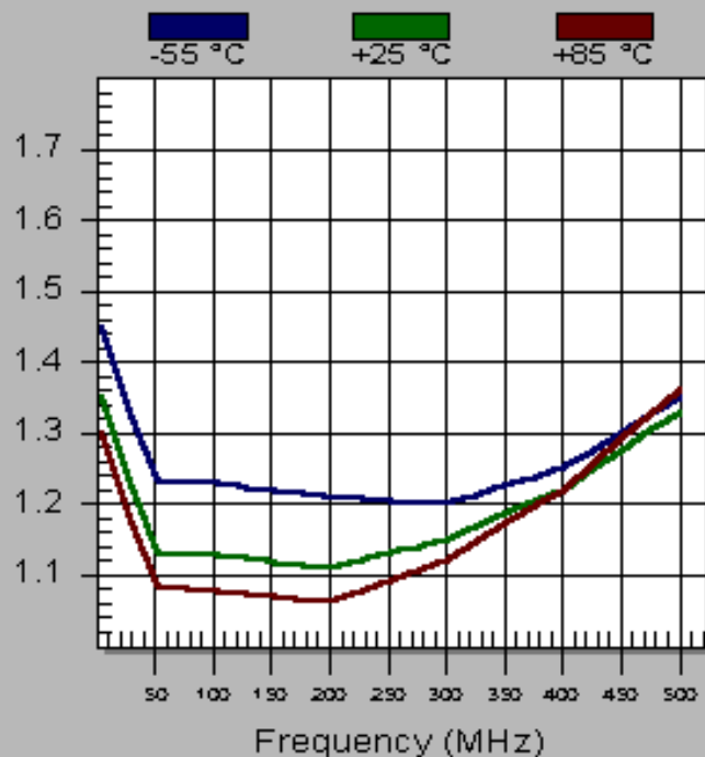
TM6520 Input VSWR
