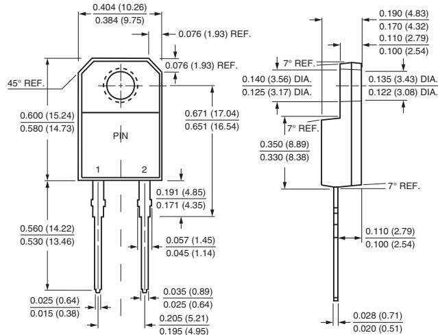
ITO-220AC
