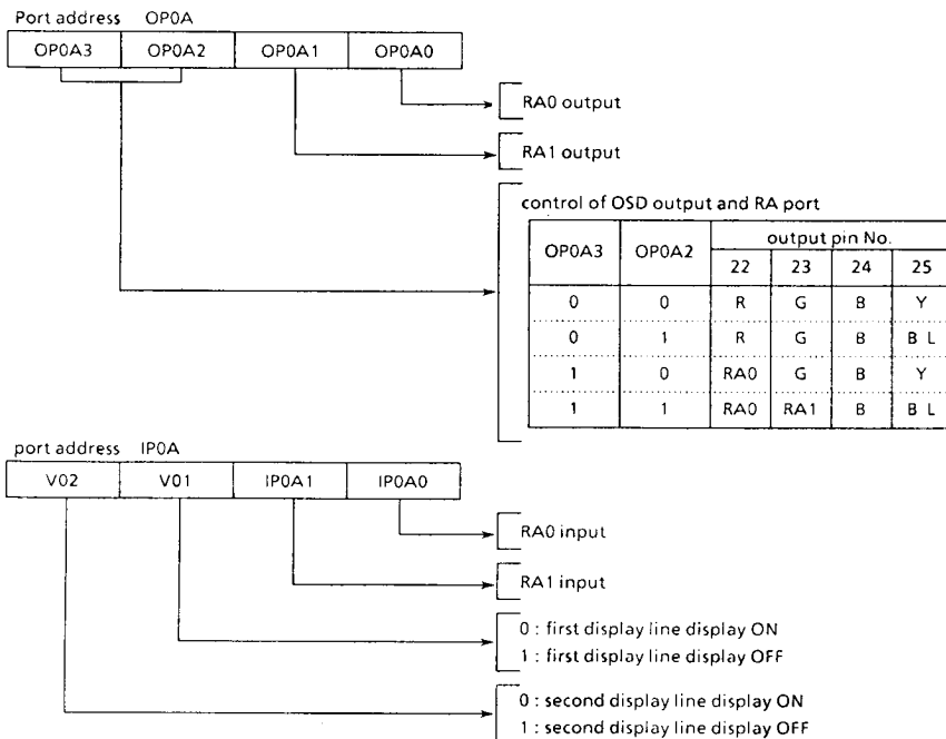
Figure 3-8. Port RA
