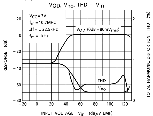
FM (IF)
