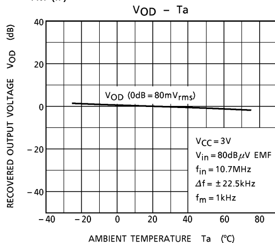
FM (IF)
