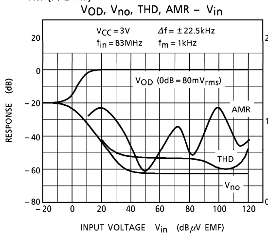
FM (IF)
