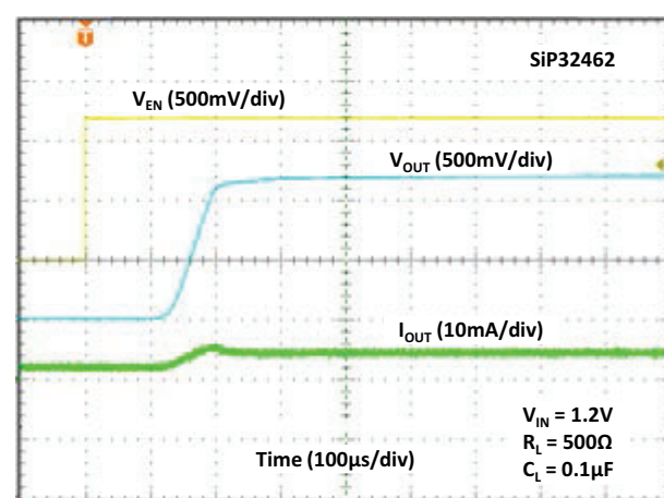
Fig. 30 - Turn-on Time
