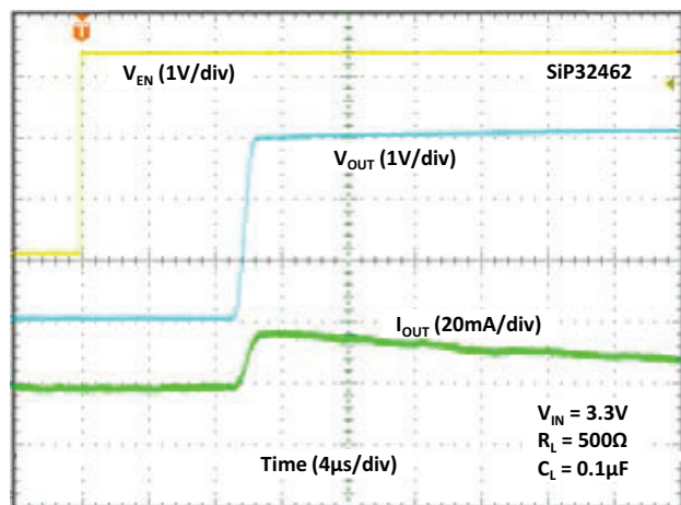
Fig. 32 - Turn-on Time
